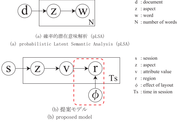
図3 pLSA と提案モデルのグラフィカルモデル Fig. 3 Graphical model of pLSA and proposed model
