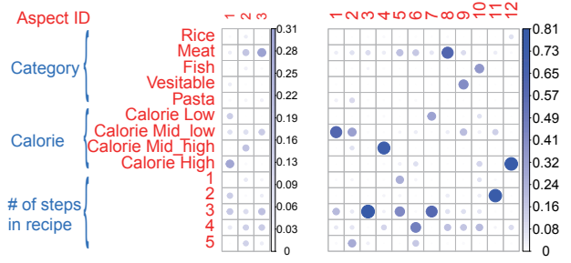
図8 学習されたアスペクトの例 ( \alpha = 0.5 , 属性: SA). 左がアスペクト数を 3 とした時の結果. 右がアスペクト数を 12 とした時の結果.
