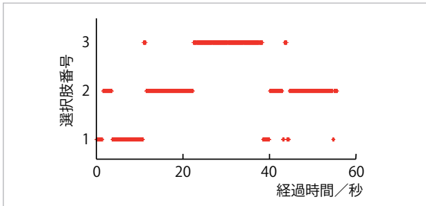
図-7 大画面端末において選択肢を閲覧する視線の滞留パターン例
